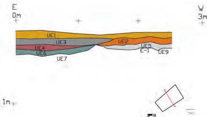
Esquema del Perfil E-O del Sondeo B (Lomo de las Viñas 1-2018)
