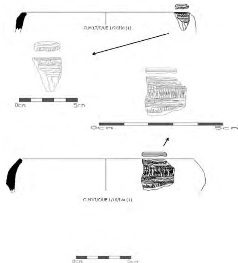
Dibujo de dos bordes cerámicos pertenecientes a las Fases III d y IVa (Sondeo c-Cueva de las Mejoras-2017)
